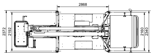
MIN. STABILISATION
